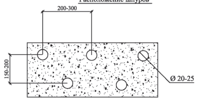
Расположение шпуров
