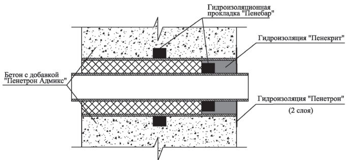
б) строящаяся конструкция
